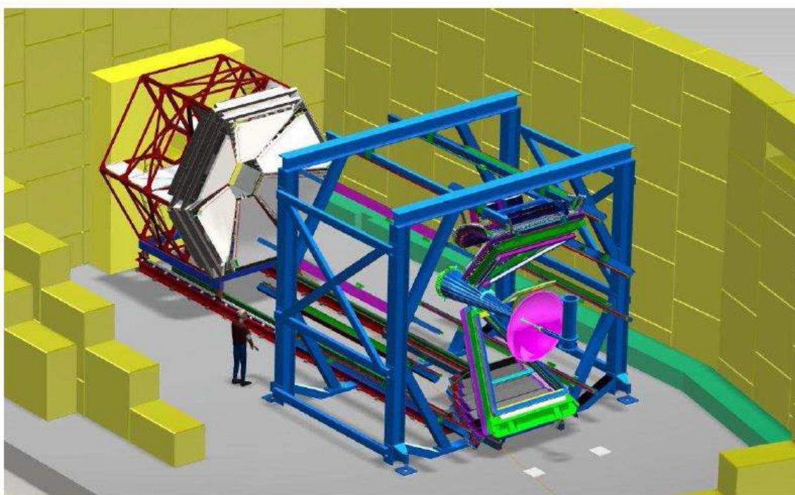
Rys.9 Poglądowy rysunek przedstawiający HADES ECAL wraz ze szkieletem głównym i detektorem HADES (dla uproszczenia pokazano tylko ramę mechaniczną detektora HADES bez jego komponentów) w hali pomiarowej w docelowym miejscu przeznaczenia (dla jasności obrazu usunięto dach oraz lewą ścianę boczną hali).
