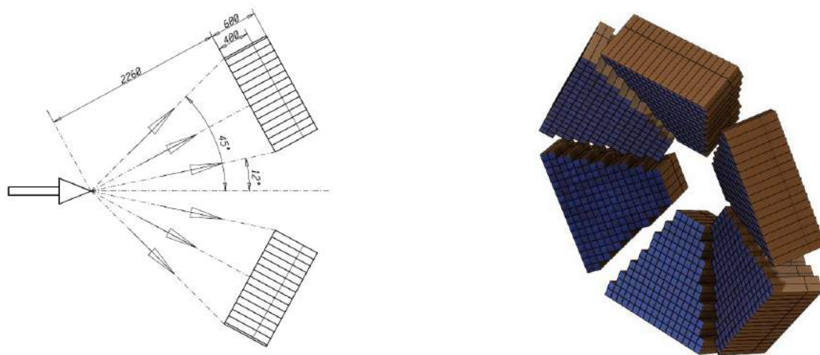
Rys.1 Lewy rysunek: Umiejscowienie modułów szkła ołowiowego kalorymetru elektromagnetycznego ECAL w stosunku do pozycji tarczy spektrometru HADES (punkt odniesienia), wymiar w mm. Prawy rysunek: Poglądowy obraz 6 sekcji kalorymetru bez Konstrukcji szkieletu głównego.
