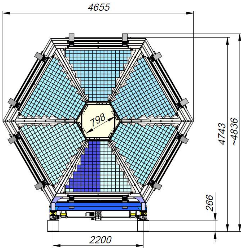
Rys2: Widok od przodu szkieletu głównego HADES ECAL z widocznymi modułami szkła ołowiowego
